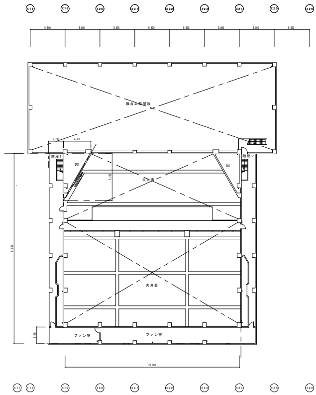
大ホール棟4階平面図 S=1/200
