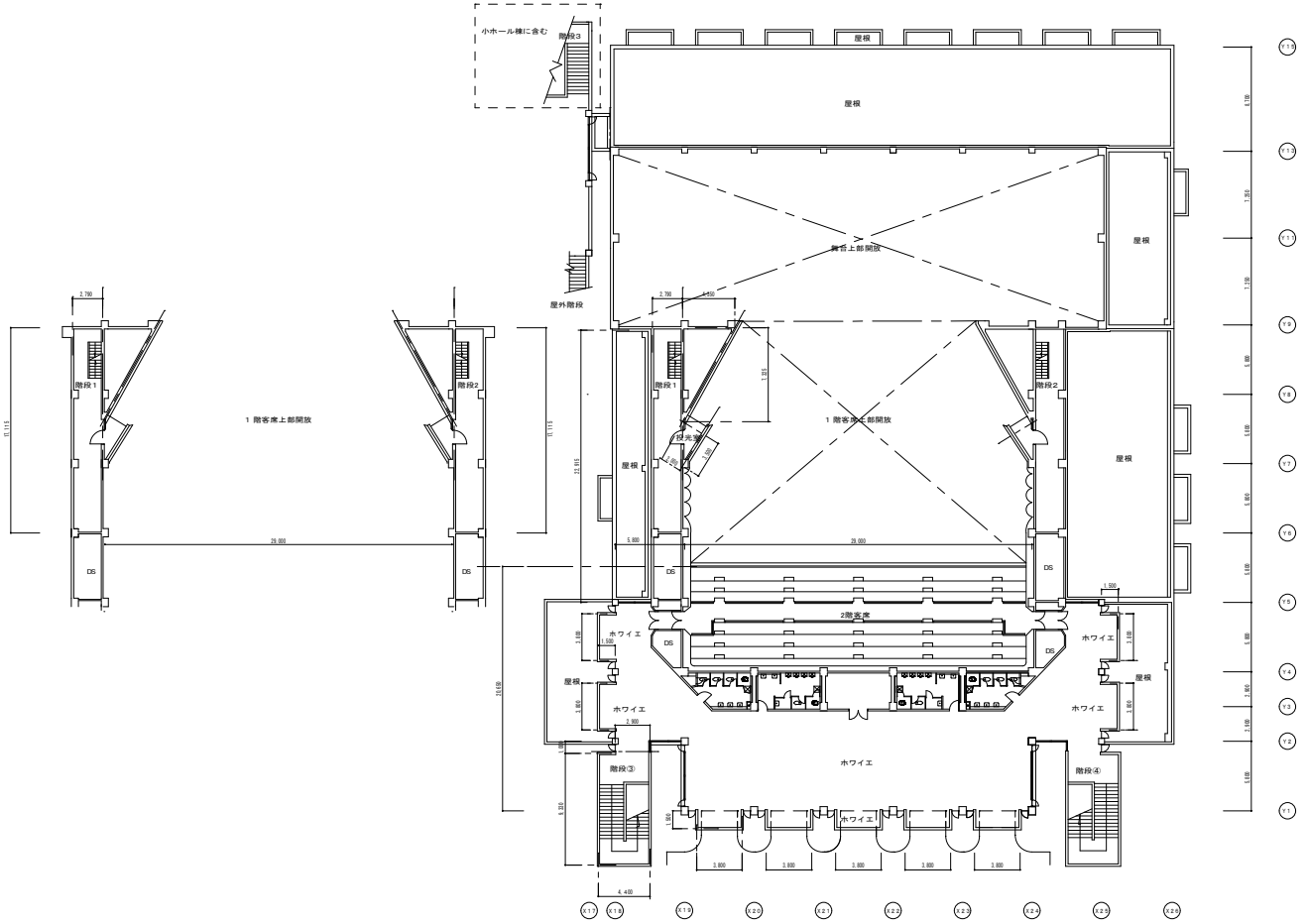
大ホール棟2階平面図 1:200
