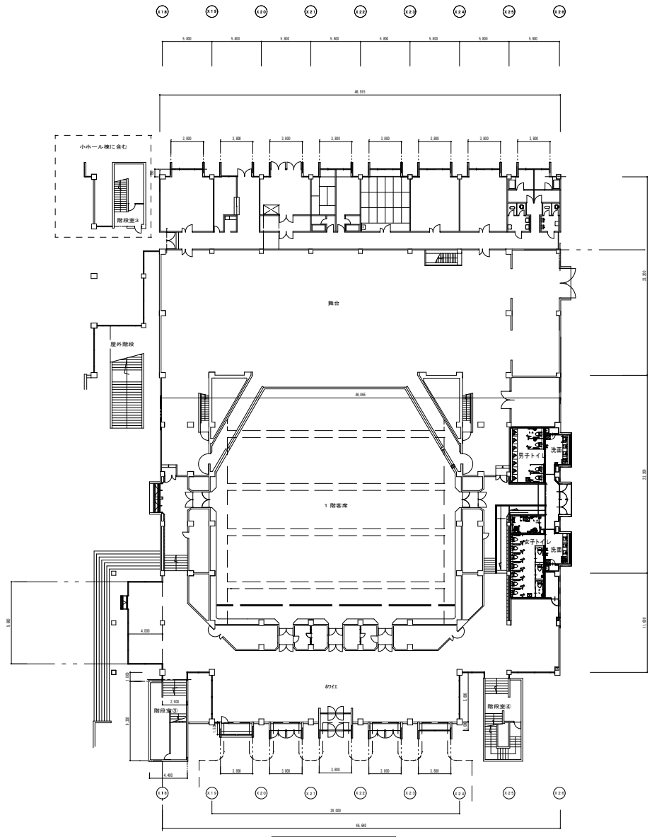
大ホール棟1階平面図 1:200
