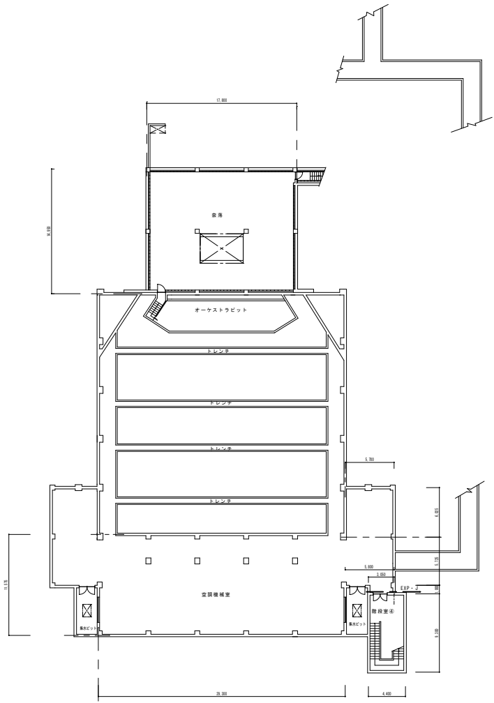
大ホール棟地下1階 平面図 1:200
