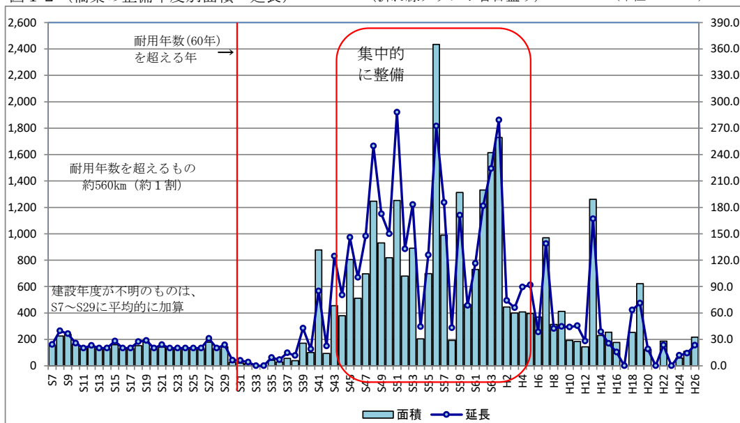
図 1 2 (橋梁の整備年度別面積・延長) (折れ線グラフ：右目盛り) (単位：㎡・m)
