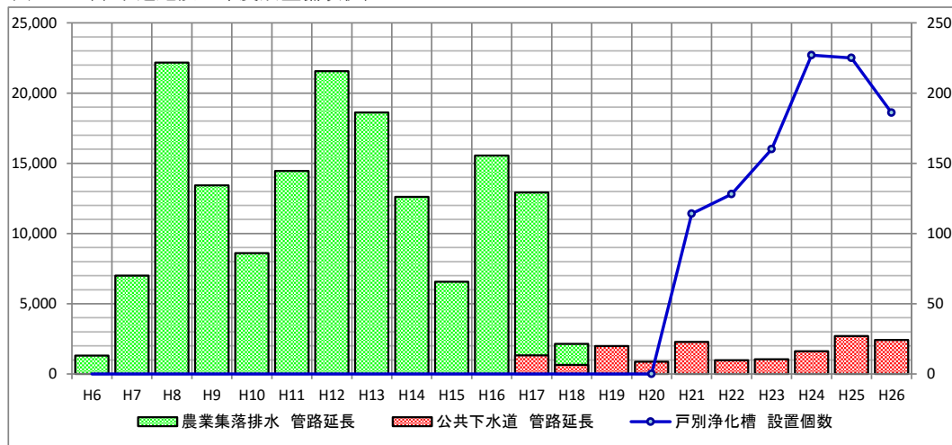
図1-3 （下水道施設の年度別整備状況） （折れ線グラフ：右目盛り） （単位：m・基）
