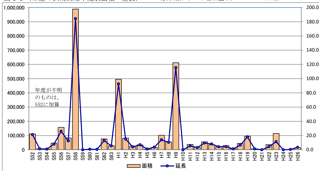
図 1 1 (市道の供用開始年度別面積・延長) (折れ線グラフ：右目盛り) (単位：㎡・km)
