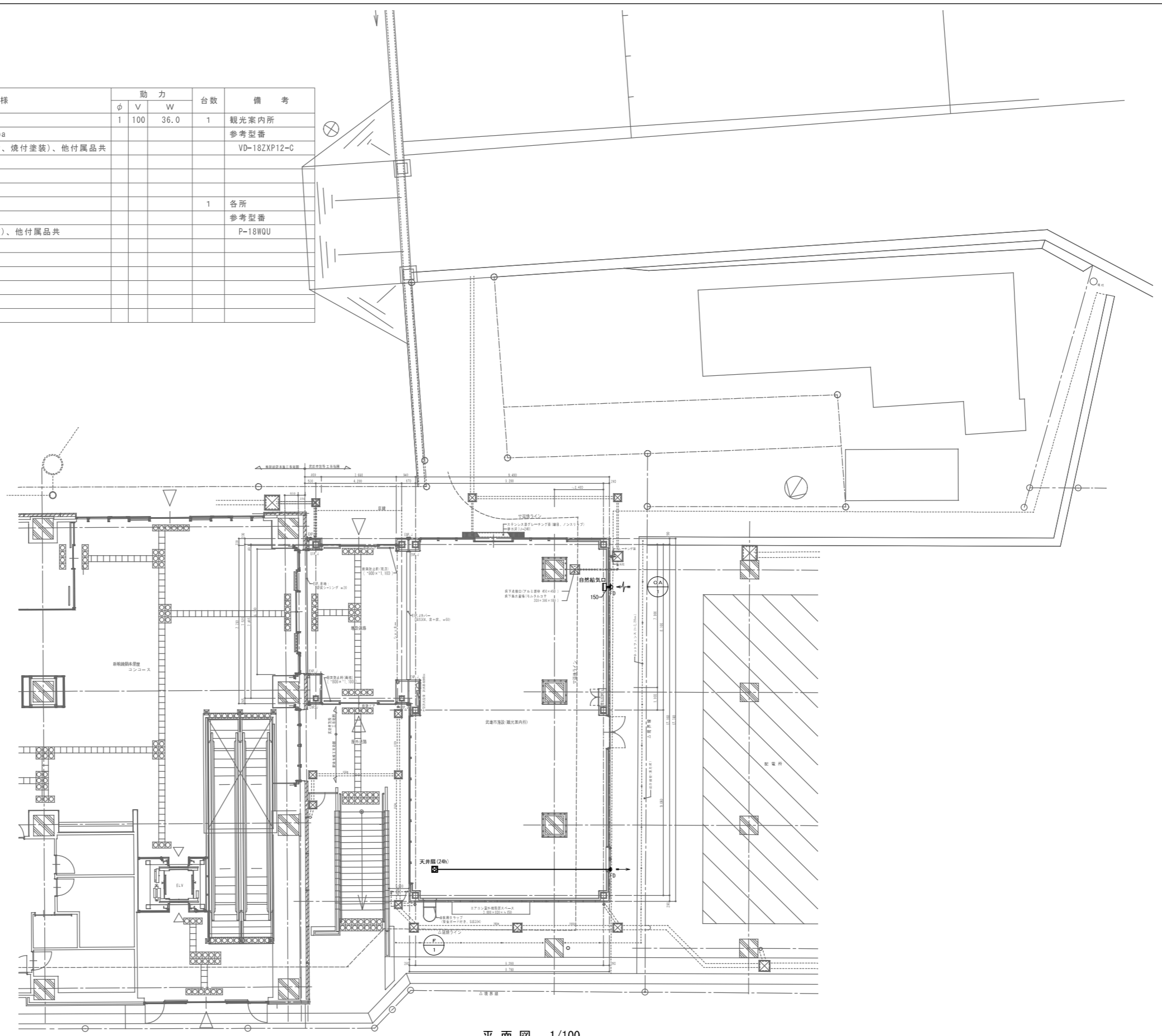
平面図 1/100
