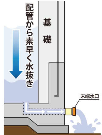
住宅基礎の水抜き設置
