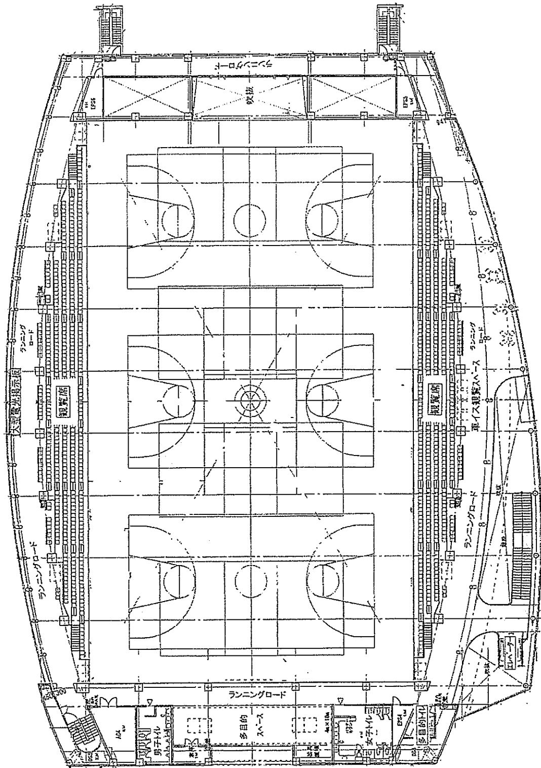
【2階平面図】
