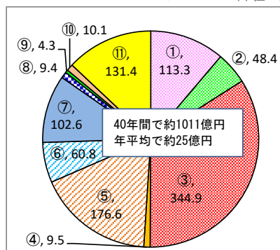
図14（建物等の更新費用）（単位：億円）
