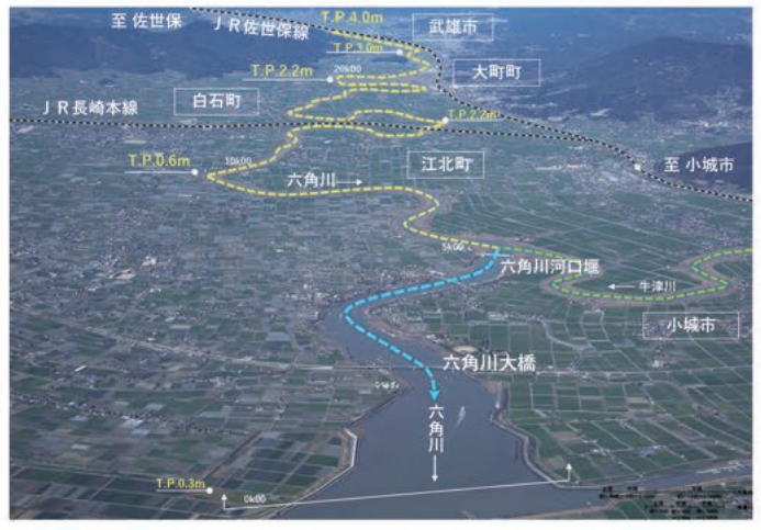
▲六角川流域は、約4割が山地、約6割が低平地
