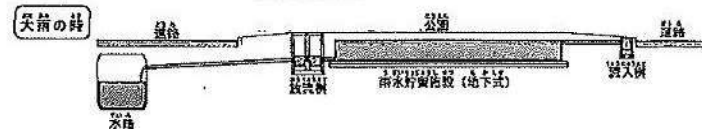
【断面図↓】
