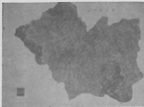
山内町地形図
