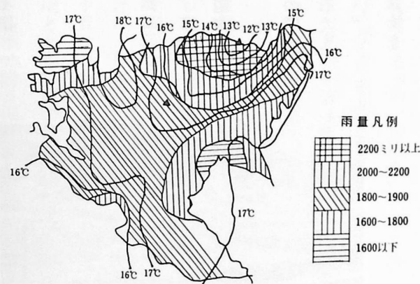
年雨量および年平均気温図
