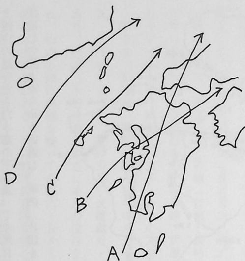
佐賀県に強い影響を与える台風のコース
